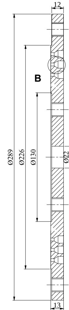
SECTION A-A
